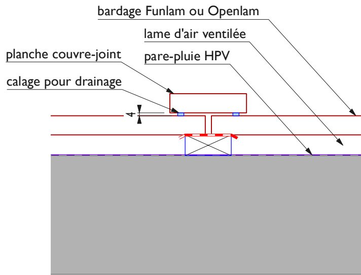
avec couvre-joint
