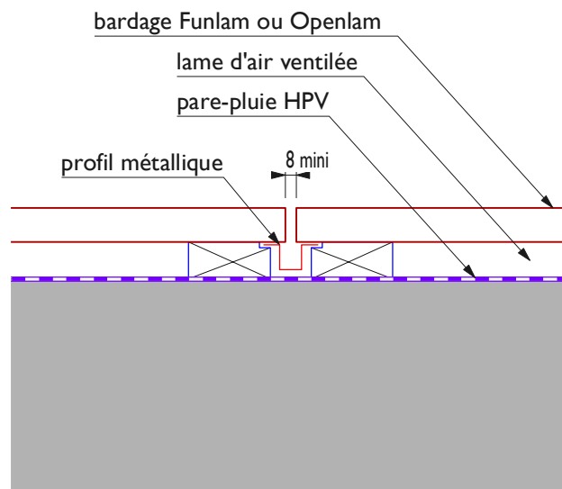
joint creux + bavette métallique
