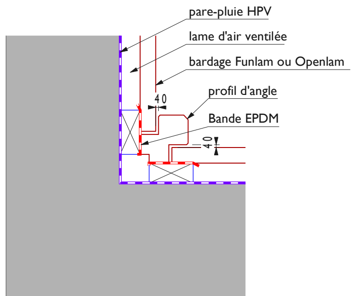
profil d'angle
